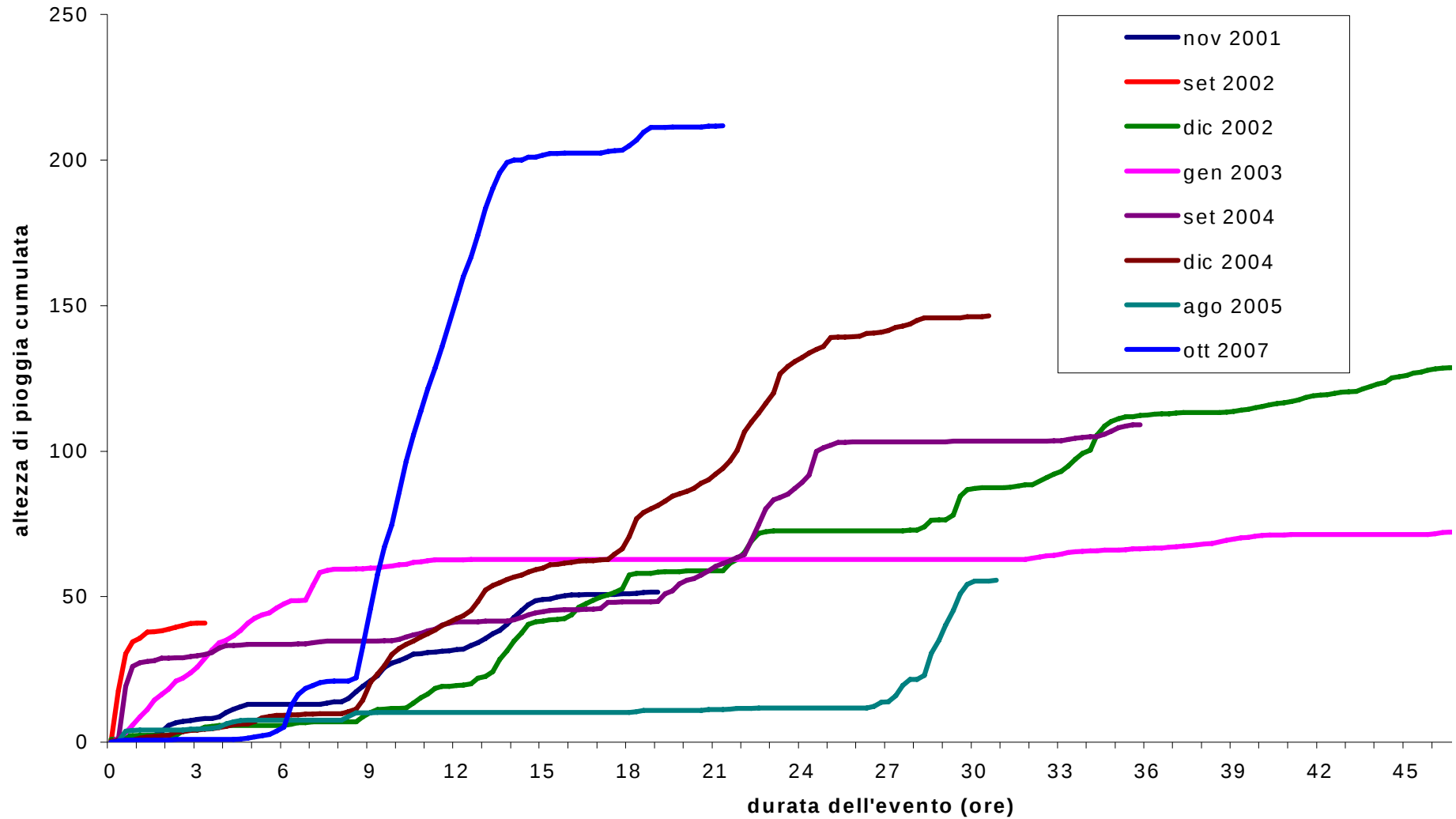
Pluviogrammi delle piogge intense relative agli anni 2001 - 2007
